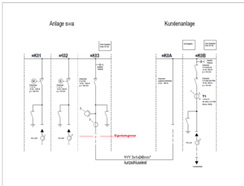
Bild 2: Beispiel für Schaltschema „Übergabestation mit Mess-/Übergabefeld mit Kabelabgang, Übergabeleistungsschalter und nachfolgendem Kundennetz“
