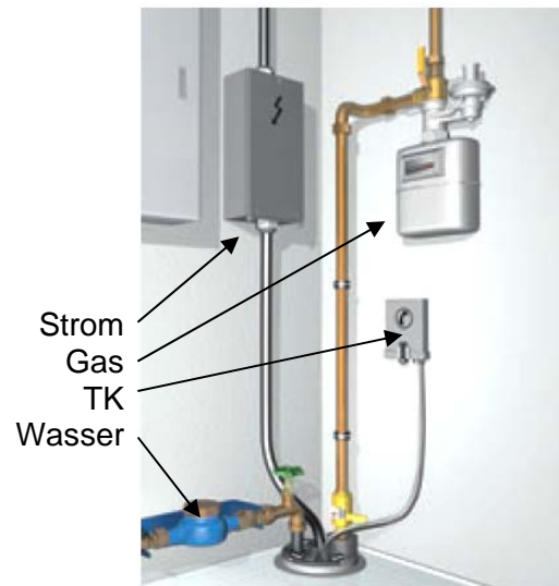
Beispieldarstellung für die Anordnung der Übergabestellen
