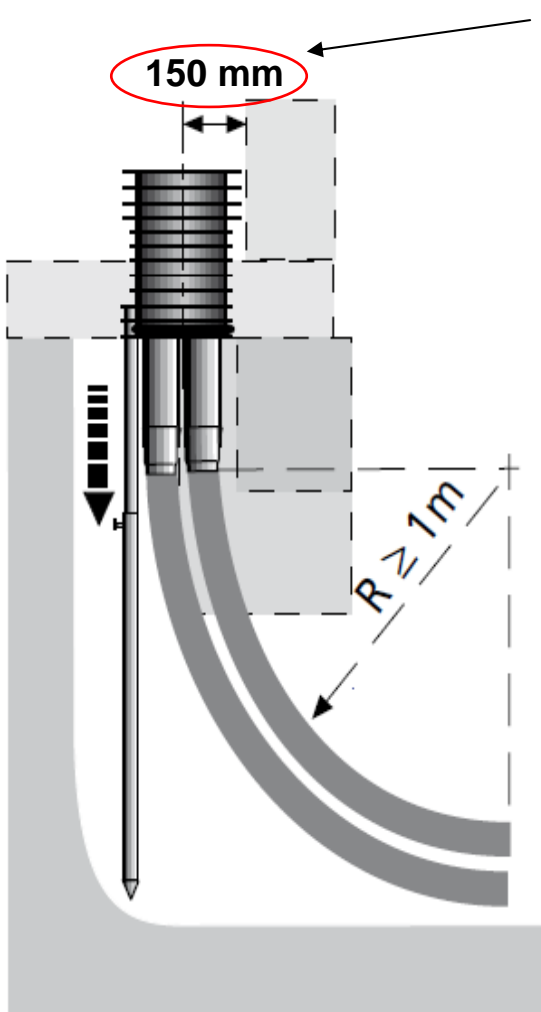
Reiheninstallation 4-fach
